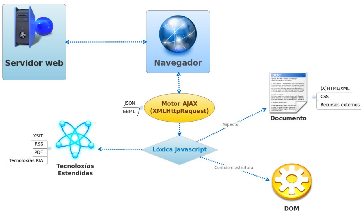
Figura 1: Funcionamento básico de AJAX.
